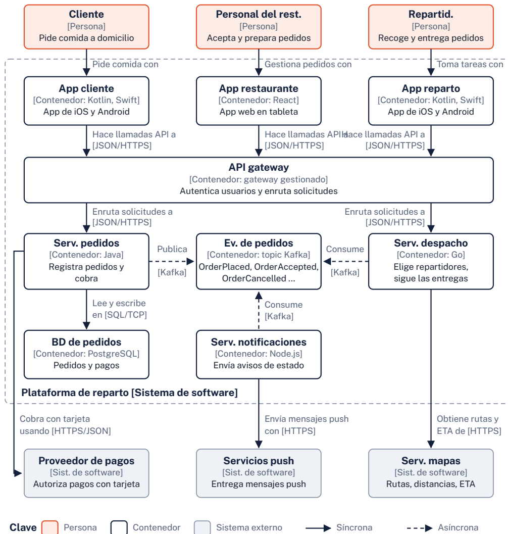
Diagrama de contenedores de la plataforma de reparto
