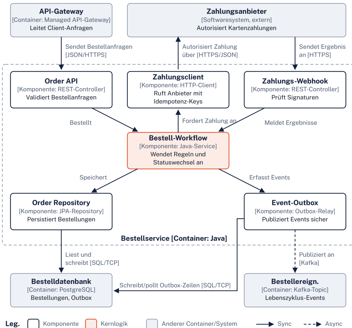
Komponentendiagramm für den Bestellservice
