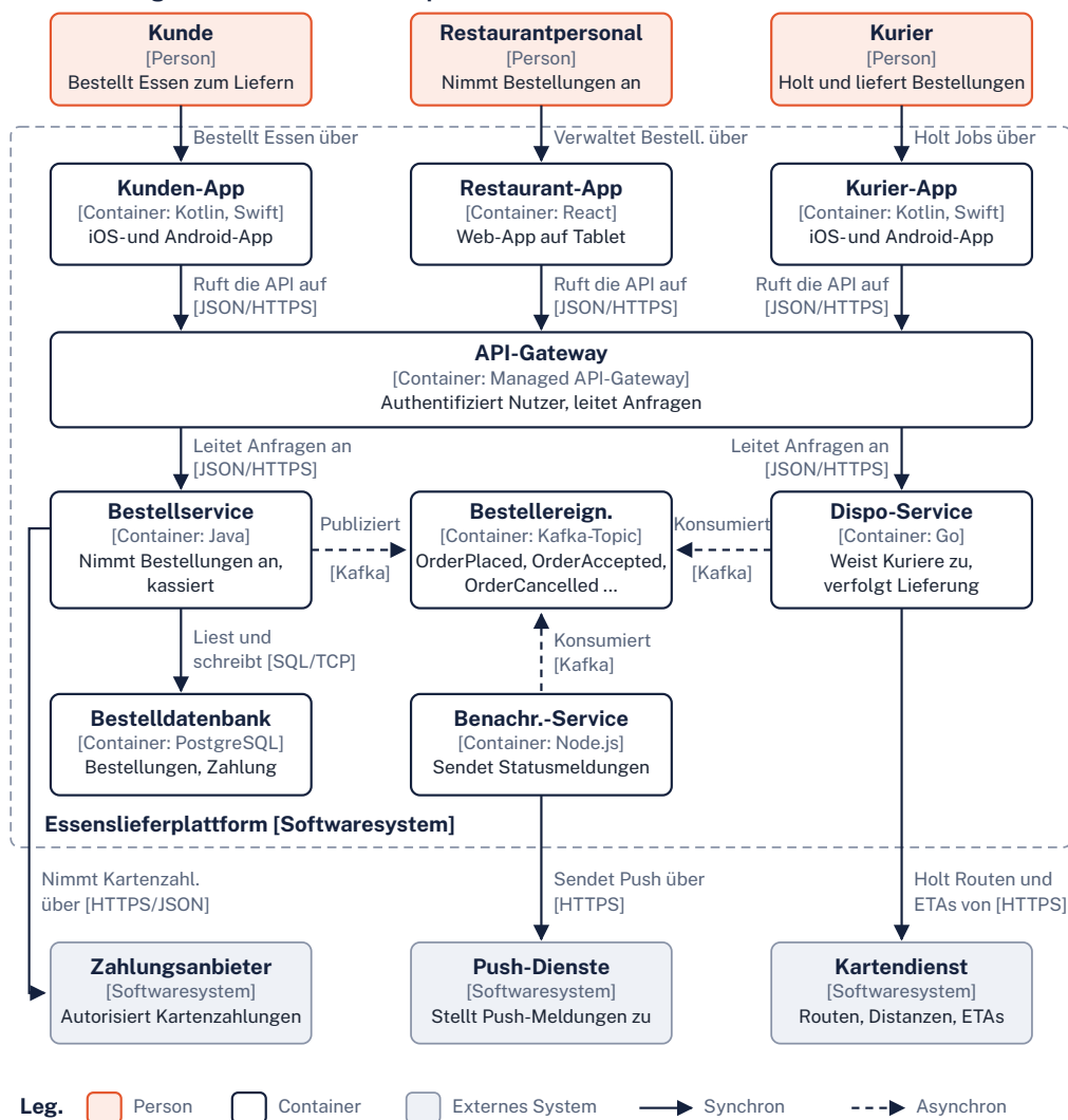
Containerdiagramm für die Essenslieferplattform
