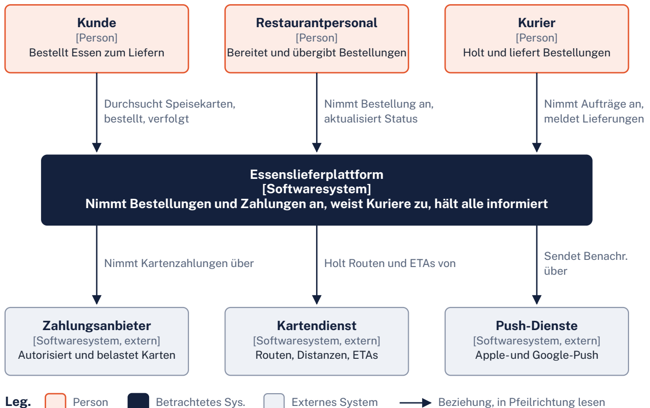
Systemkontextdiagramm für die Essenslieferplattform
